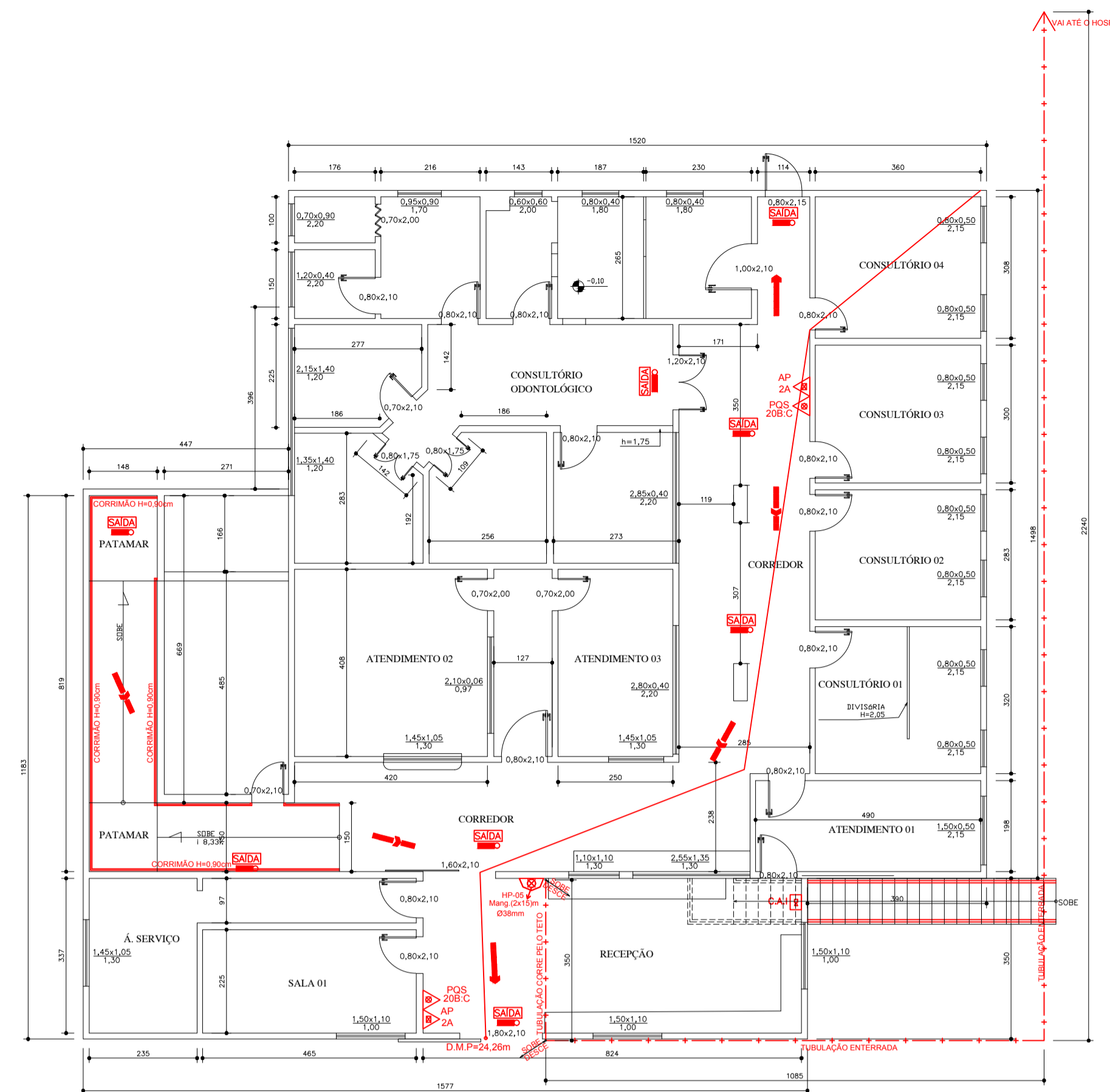
1 PLANTA BAIXA- TÉRREO - POSTO SAÚDE ESCALA 1:100 ÁREA 320,79M2
