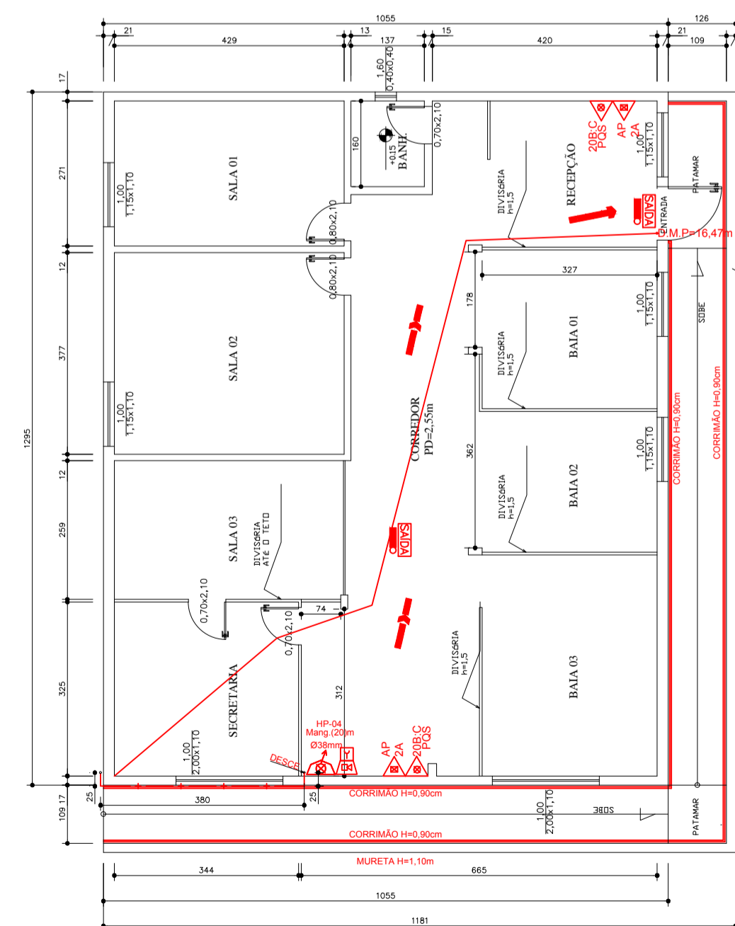
4 PLANTA BAIXA- 1º PAVIMENTO- SEC. SAÚDE ESCALA 1:100 ÁREA 136,47M2
