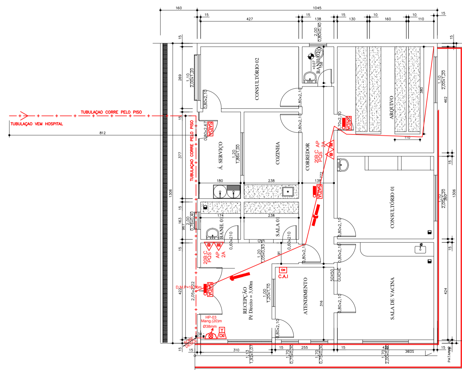
3 PLANTA BAIXA- TERREO - SEC. SAÚDE ESCALA 1:100 ÁREA 136,47M2
