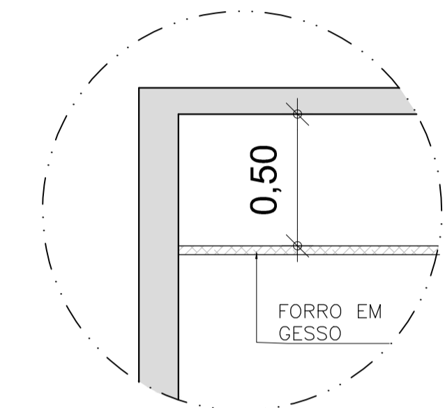
DETALHE 01 ESC: 1/20
